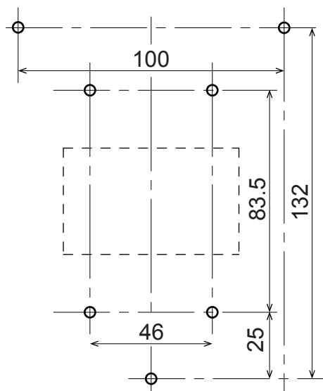
図4 取付寸法図
