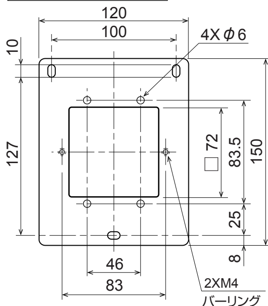
図6 補助プレート寸法図
