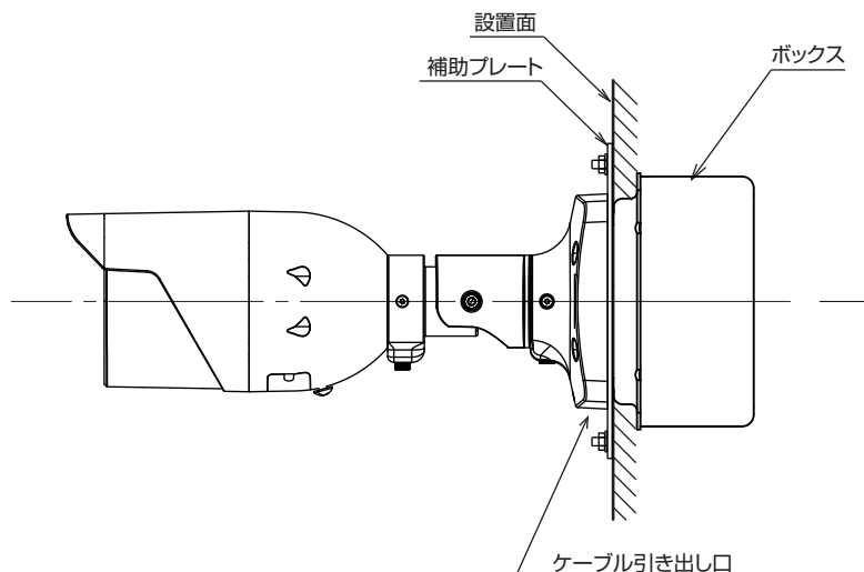
図5 ボックス施工例
